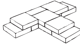
Hiladas pares 2,4,6 ...
