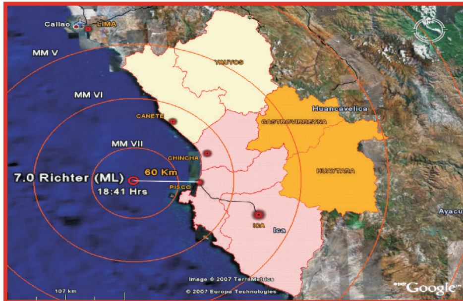
“Epicentro del sismo de Ica 2007”.
