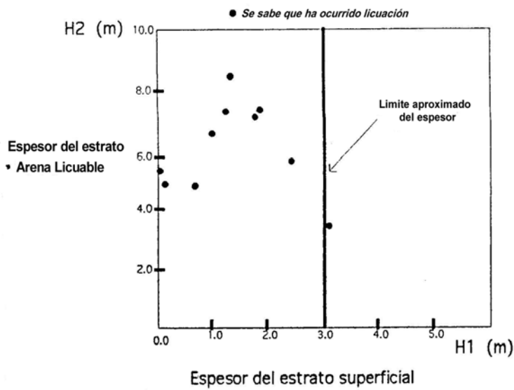
EFEECTO DEL ESTRATO SUPERFICIAL EN LAS CAUSAS DE MANIFESTACION SUPERFICIAL DE LICUACION (Ishihara, 1978) (a)
