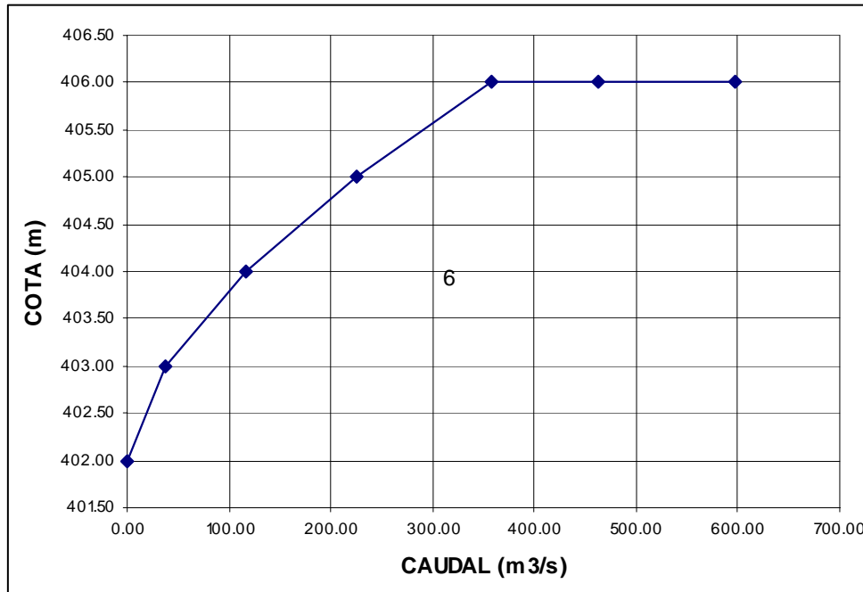
GRAFICO N° 12: Curva de Gasto Sección 36+100
